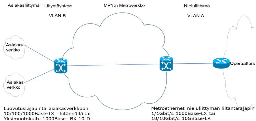
Kuva 1. Metroethernet-yhteyksien toteutus
