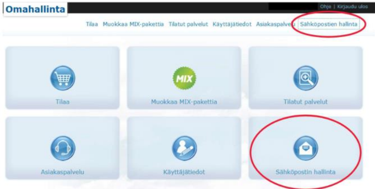
Kuva 5. salasanan vaihto
